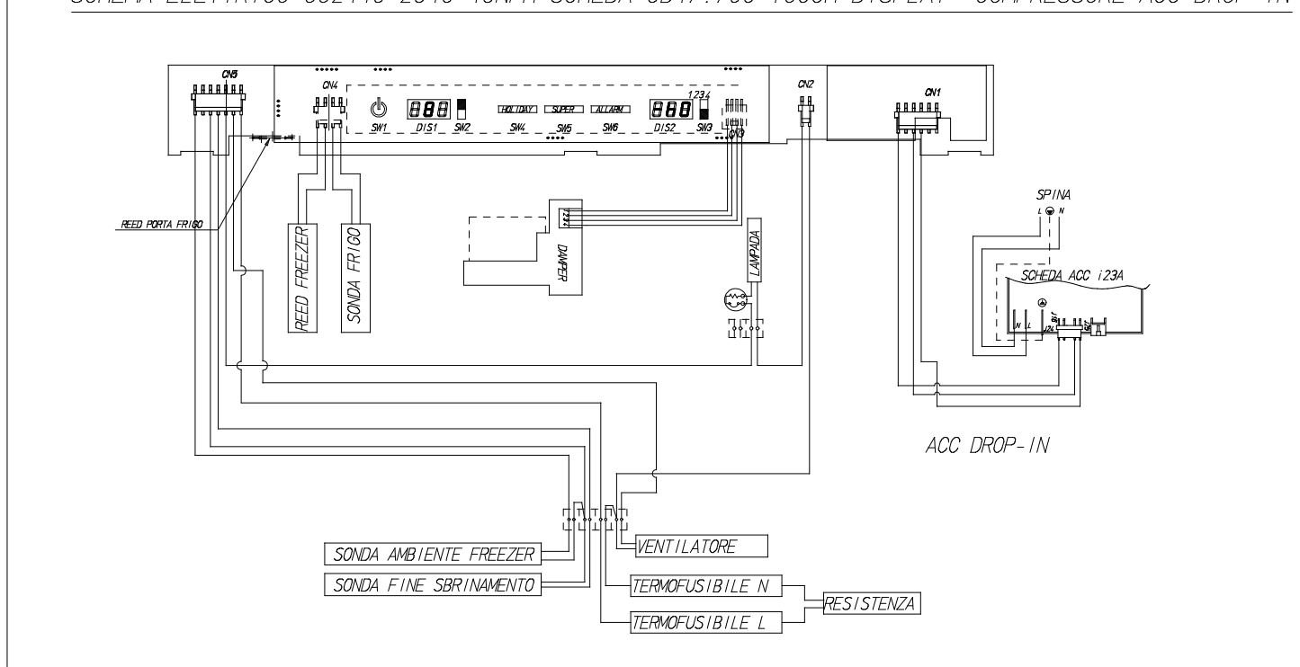
SCHEMA ELETTRICO GO2110-2510-43NFH SCHEDA CB17.700 TOUCH DISPLAY COMPRESSORE ACC DROP-IN
