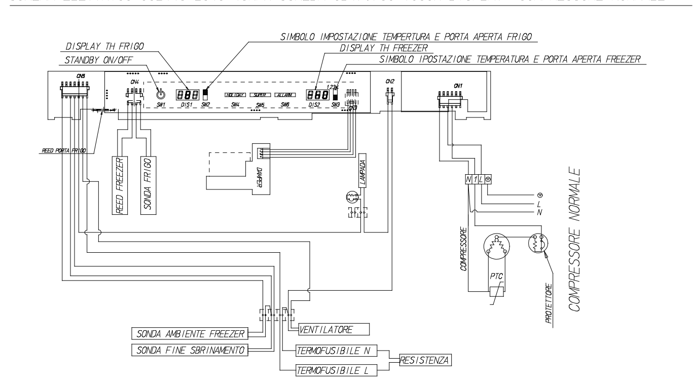
SCHEMA ELETTRICO GO2110-2510-43NFH SCHEDA CB17.700 TOUCH DISPLAY COMPRESSORE NORMALE
